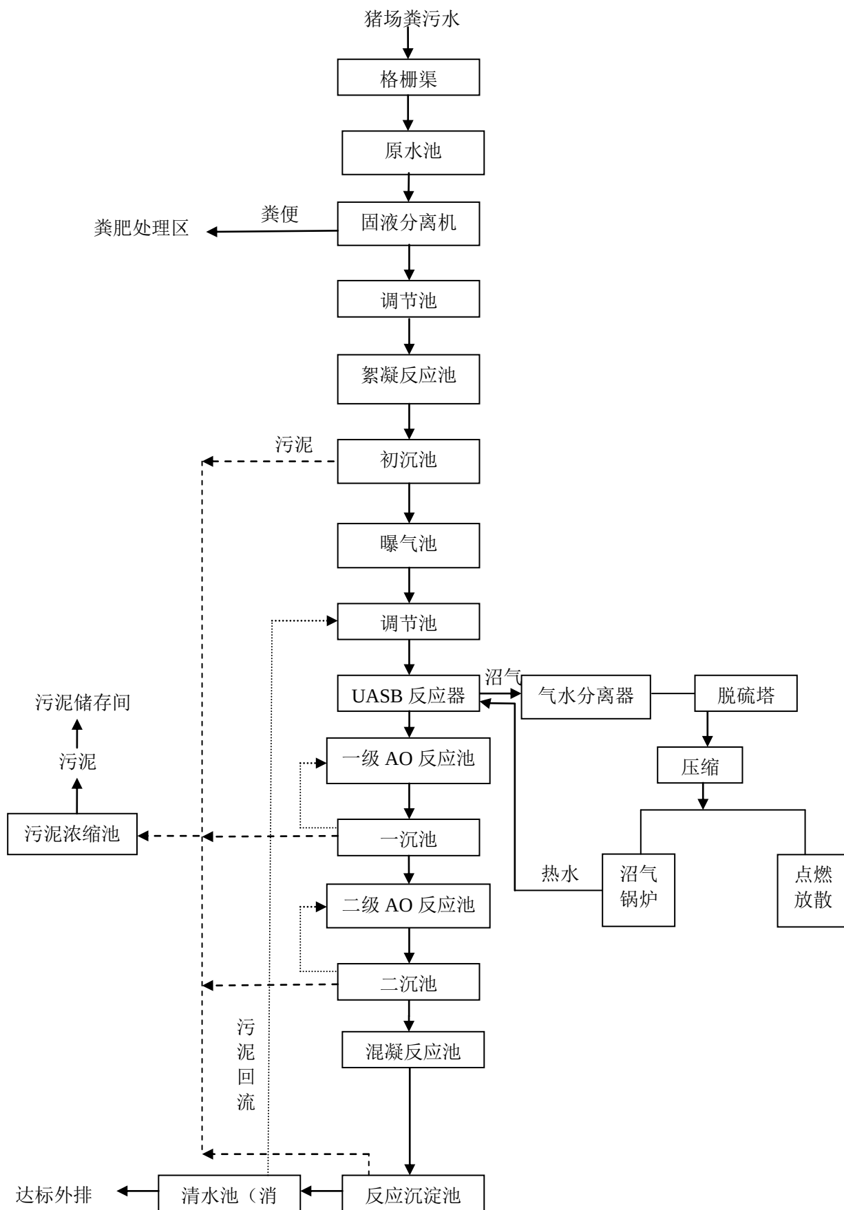
图 8.2.2-1 污水处理工艺流程图
