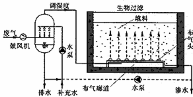
图 7.2-1 生物除臭塔除臭工艺流程
