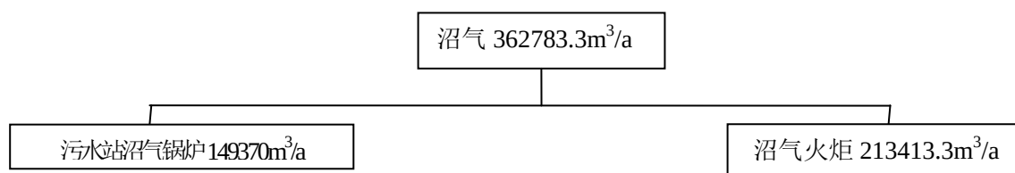
图 8.2.2-2 工程沼气平衡图
